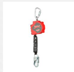
MM-3100431 Auto Retrácil de Cinta con Gancho Giratorio Pequeño de Acero y Mosquetón 6.1 M
